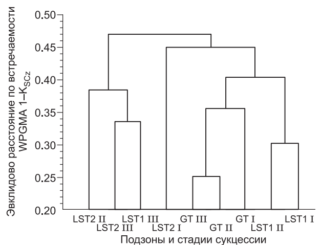
Рис. 6. Дендрограмма сходства флористических списков по стадиям сукцессии и природно-климатическим зонам. Подзоны: LST1 – северная лесостепь; LST2 – южная лесостепь; GT – горно-таежная подзона. I, II, III – стадии растительной сукцессии.
